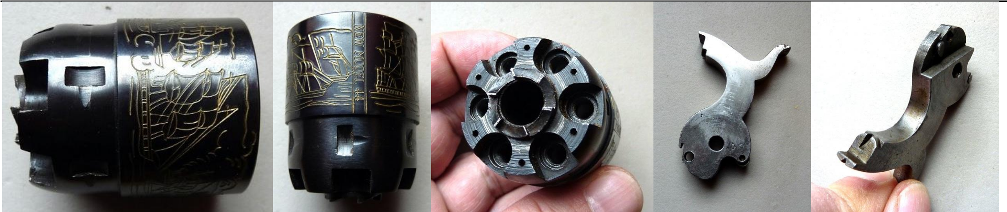
Frankenstein RNMA cylinder: gold inlaid cylinder engraving; no digits of S/N on cylinder & no safety pins; hammer: w/o S/N, could have been milled from a solid not cast | Frankenstein-RNMA Trommel: mit Gold eingelegter Gravur ohne S/N & ohne Sicherungsstifte; Hammer: ohne S/N, könnte aus dem Vollen gefräst sein, kein Gussteil
